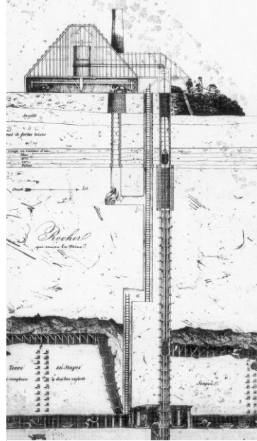
Détail d'une gravure publiée à Douai dans la première moitié du XIX ème siècle sous le titre "Idée d'une exploitation de la mine de houille". crédit : Centre Historique Minier
