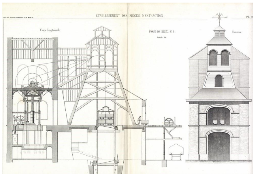
Coupe transversale de la fosse Villars à Denain in Amédée Burat, Le matériel des Houillères en France et en Belgique : atlas descriptif des appareils, machines et constructions employés pour exploiter la houille, 1860 - crédit : Centre Historique Minier (prêt ANMT)
